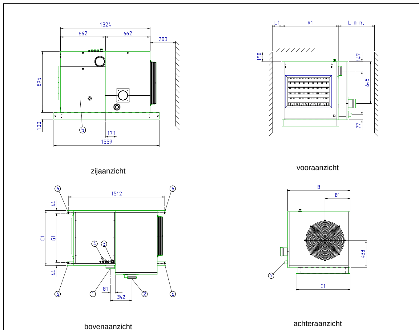
Figuur 1 : AFMETINGEN
