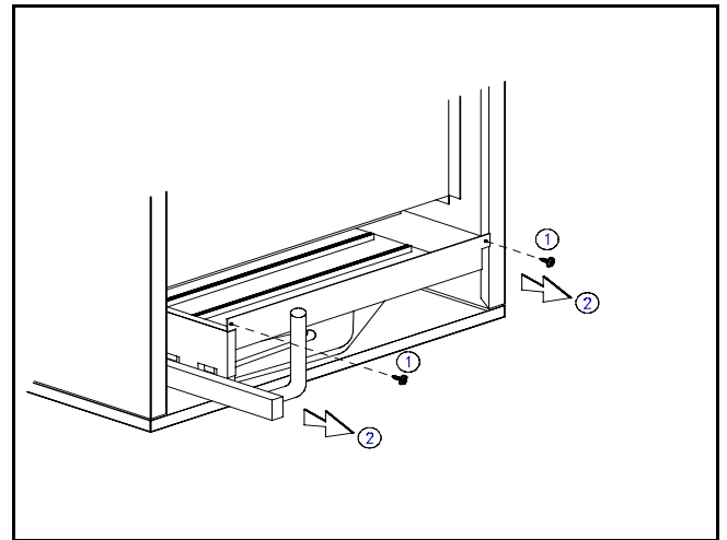
Figuur 12 : VERWIJDEREN BRANDERREK
