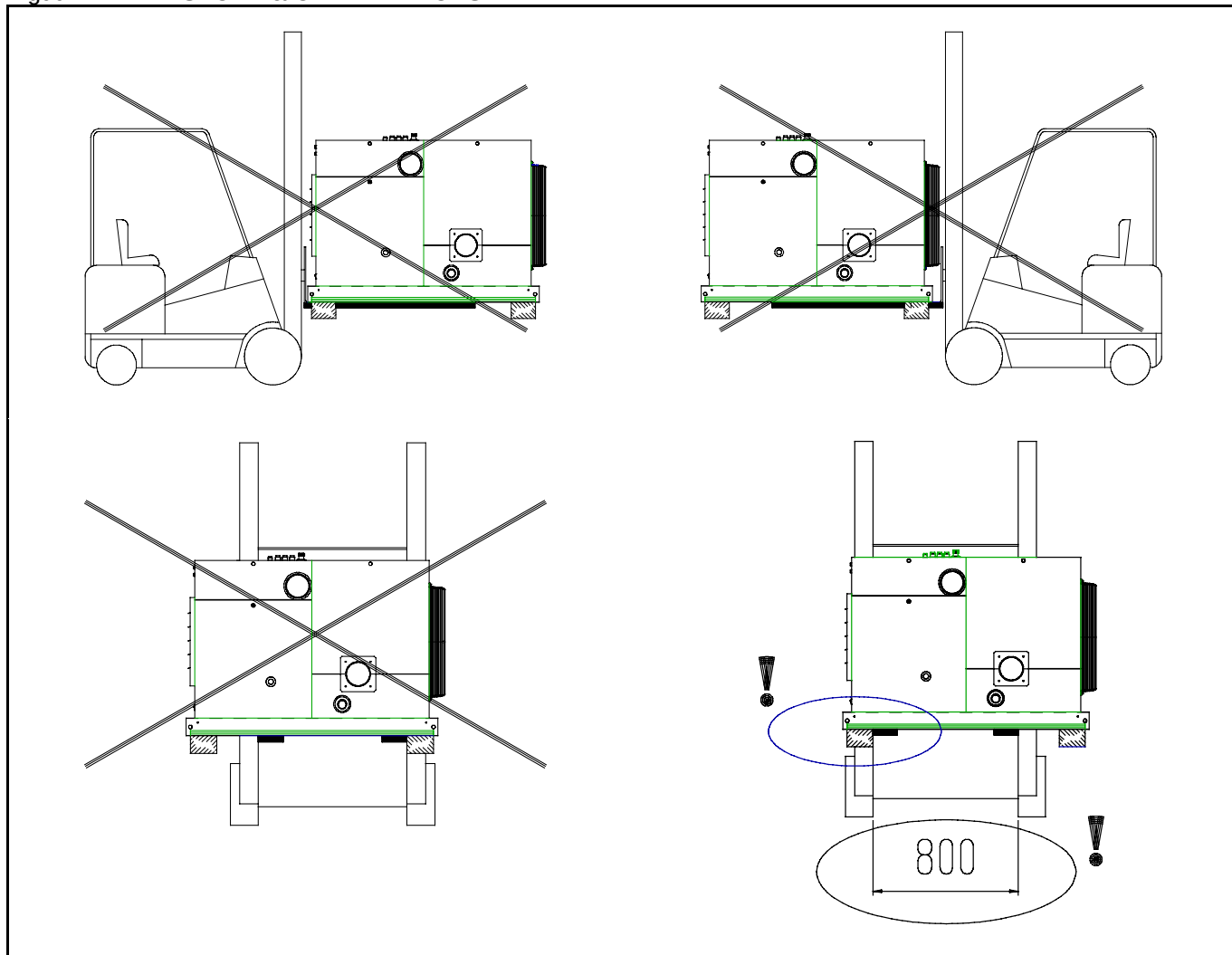
Figuur 2 : TRANSPORT & OPTILLEN TOESTEL
